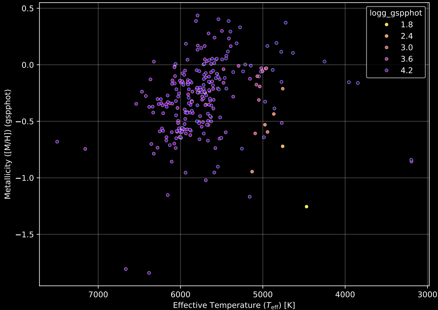
GALAH DR4 Field: [211] Stellar Population Parameters (n= 257)
