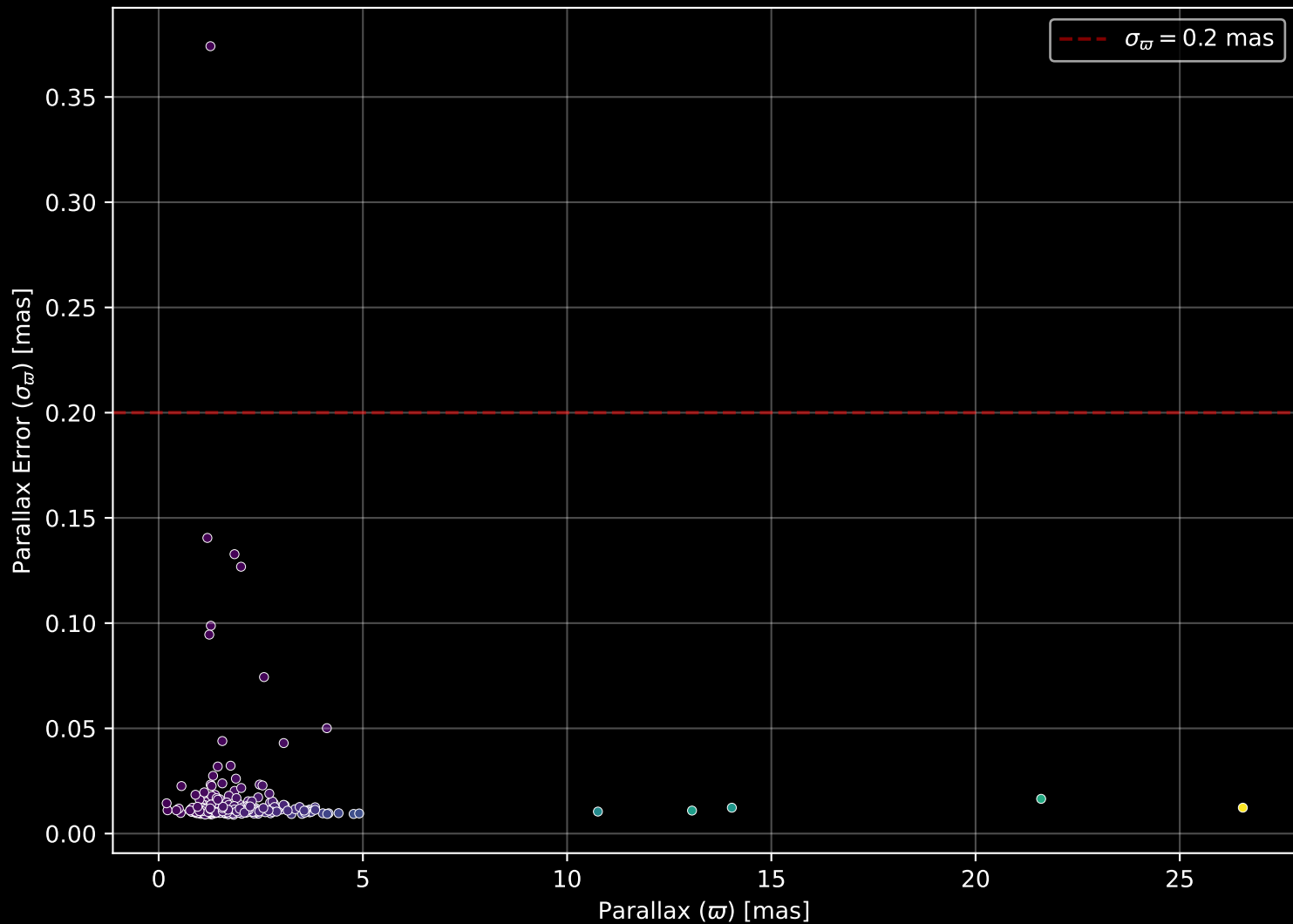
GALAH DR4 Field: [211] Parallax Quality (n= 257)
