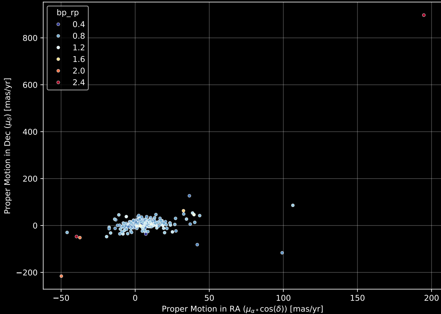
GALAH DR4 Field: [211] Proper Motion Diagram (n= 257)
