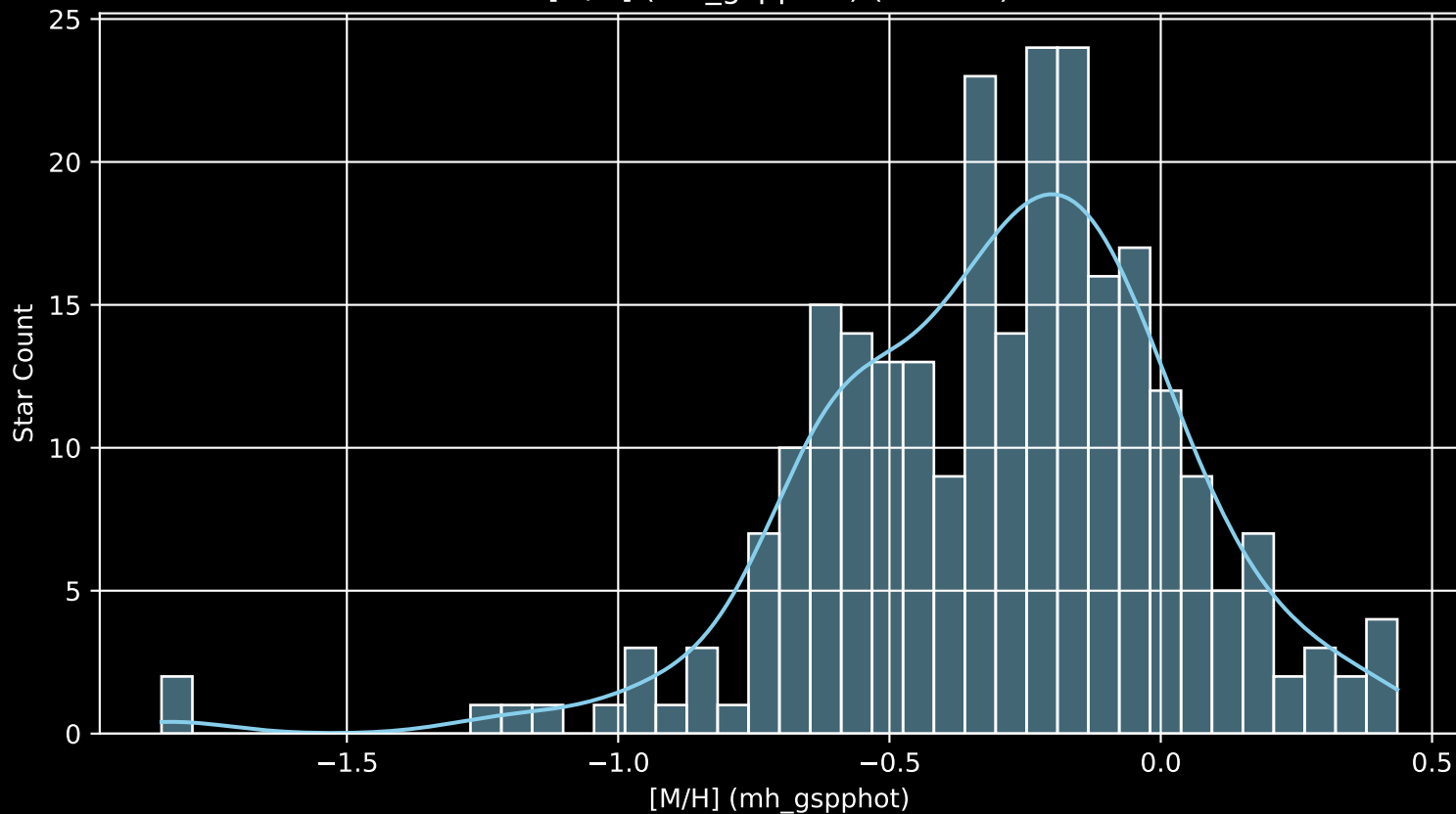
GALAH DR4 Field: [211] [M/H] (mh_gspphot) (n= 257)
